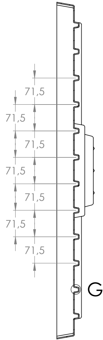
SECTION D-D
